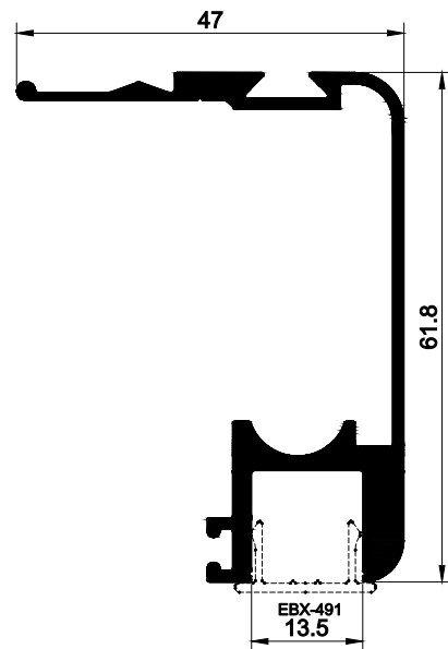
EVT-007 0,895 kg/m
