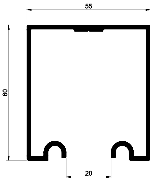
EBX-280 0,510 kg/m
