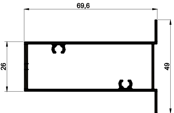
E90-586 0,577 kg/m
