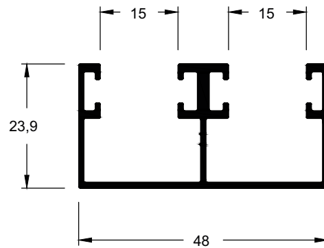
EVT-028 0,515 kg/m
