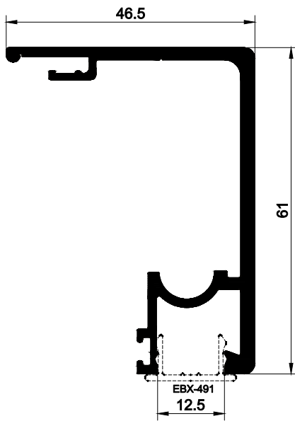
EBX-035 0,967 kg/m
