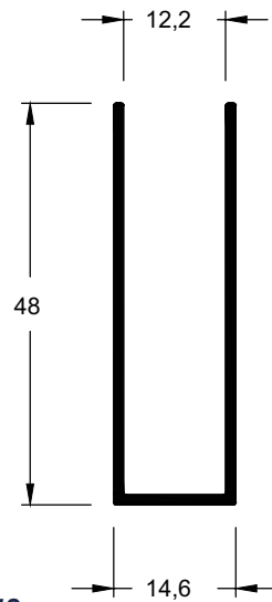
EPU-555 0,170 kg/m
