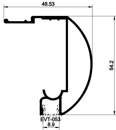
EBX-107 0,545 kg/m
