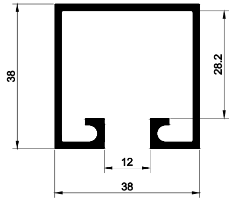
EPO-990 0,751 kg/m
